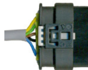
Рис. 3. Фиксатор закрыт.
